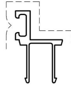
CF432 35mm DOOR STOP
